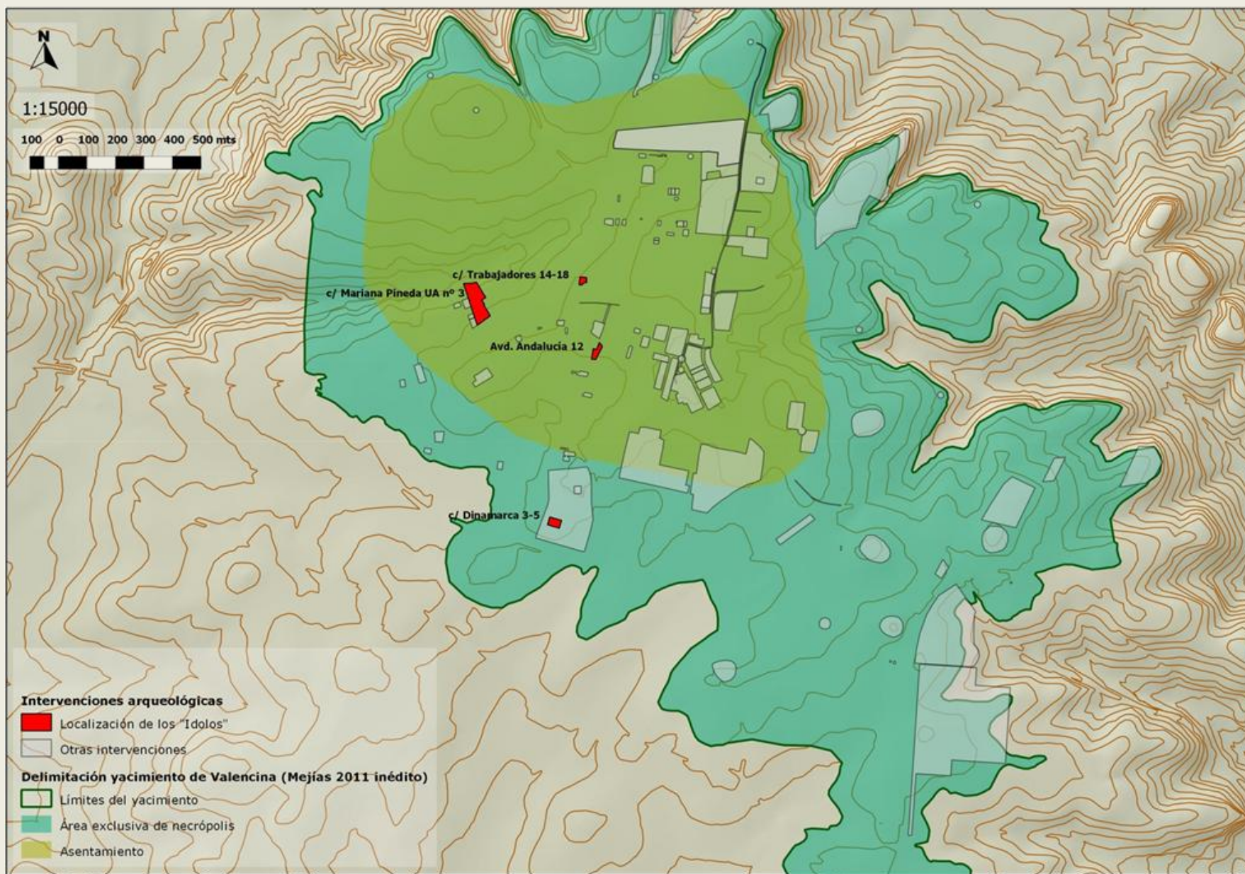
Fig. 1.— Delimitación del yacimiento y localización de los hallazgos (fuente Juan Carlos Mejías García)
