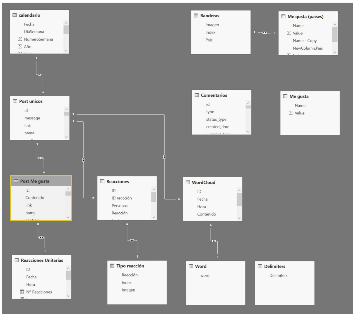
Gráfico 3. Relaciones entre las tablas para la elaboración del cuadro de mandos de Facebook
