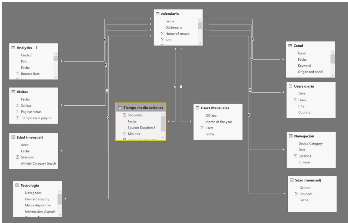
Gráfico 1. Diseño relacional de tablas.
