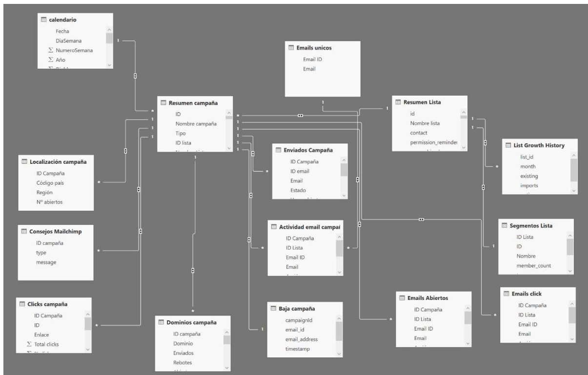
Gráfico 5. Relaciones entre tablas Mailchimp.
