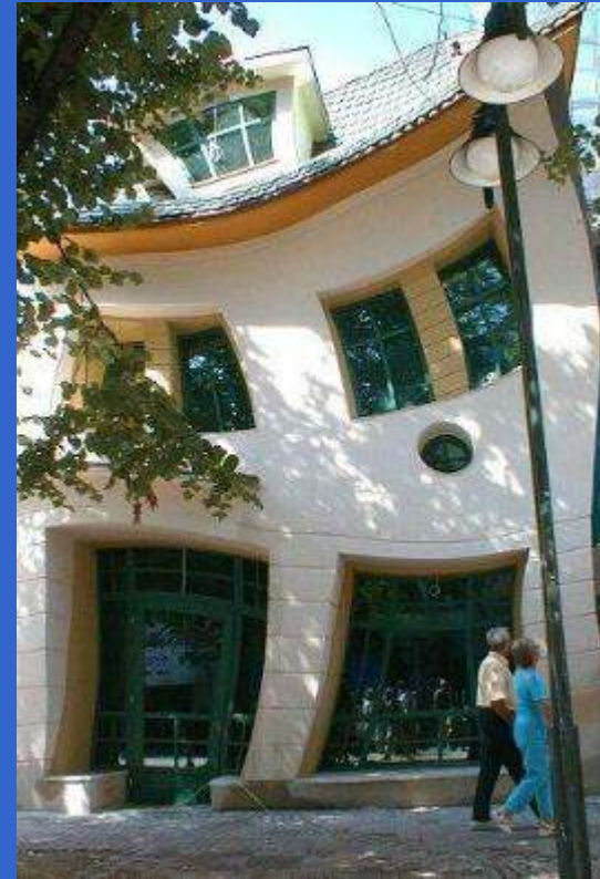
Deformación Topológica
